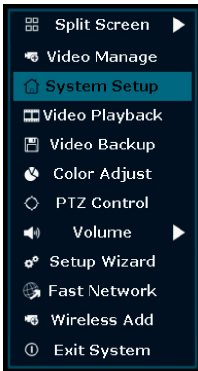
8: Menuoverzicht
