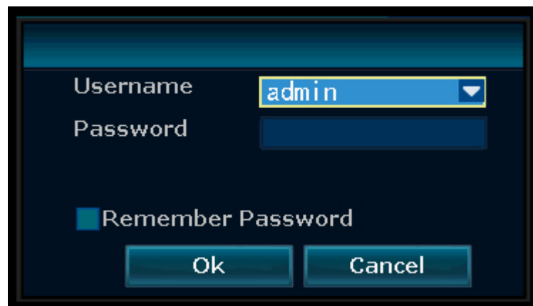
Abb. 3: Anmeldung
